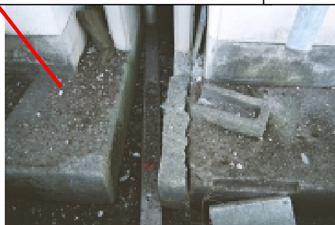
写真 22 2 棟の連結部分の損傷
