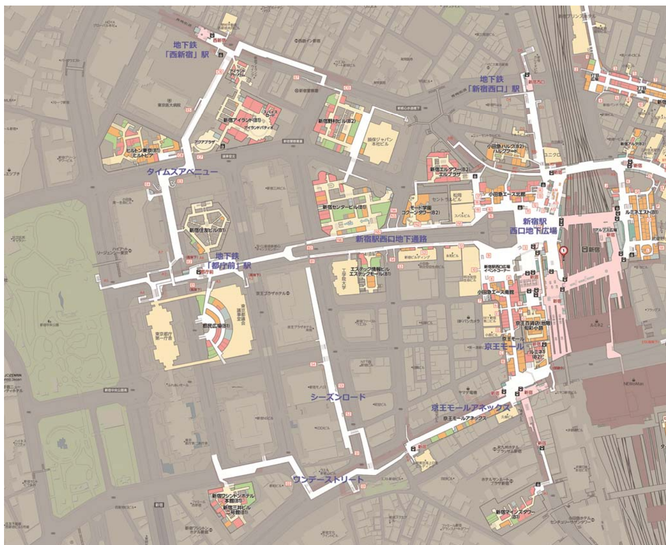
図 1 新宿駅西口地下街配置構成図（Yahoo!地図を元に著者作成）
