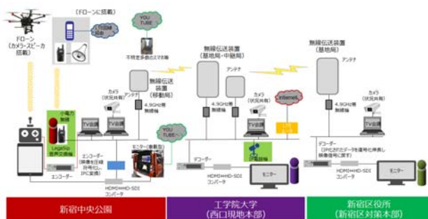
図 2 各拠点における機器類の接続構成と実験環境
