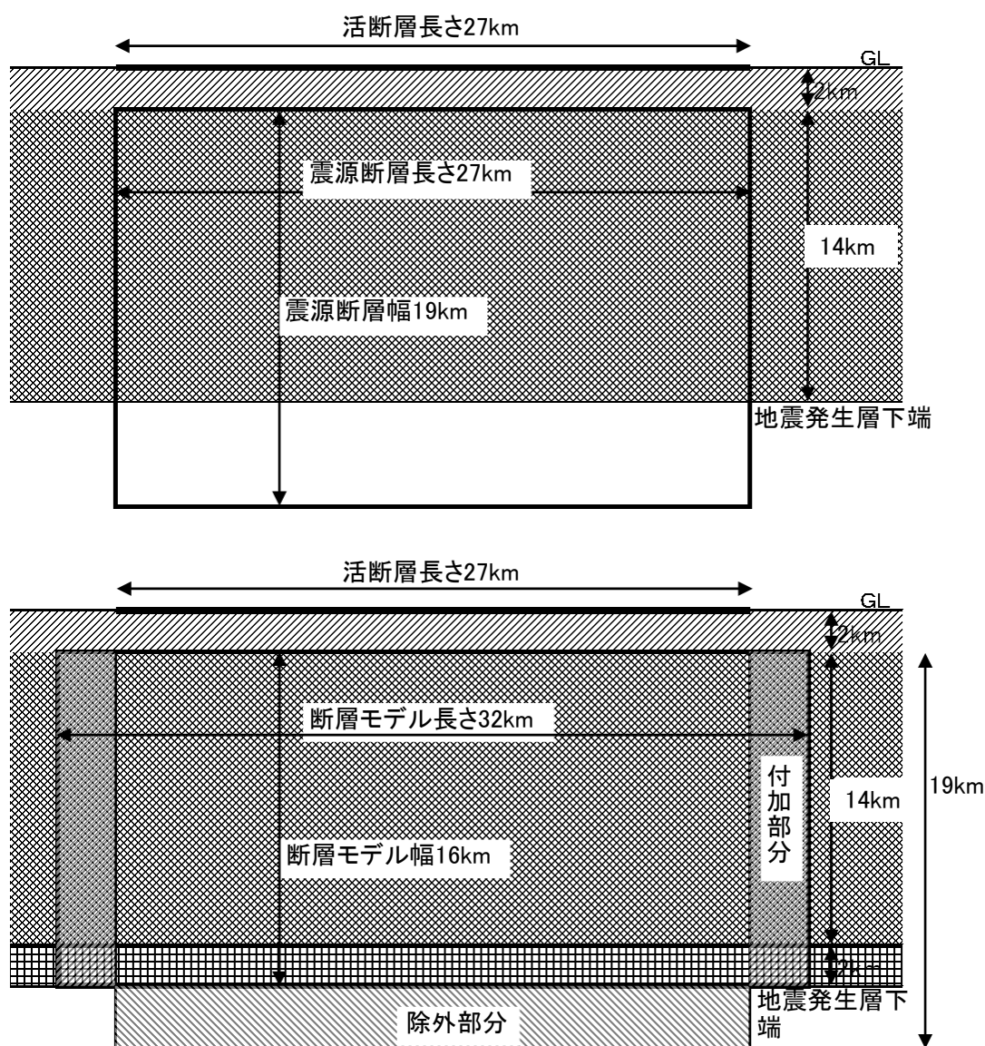
断層モデル長さおよび幅の概念図
