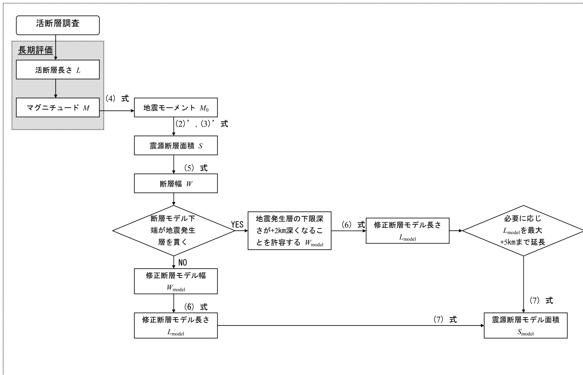
付図3 活断層で発生する地震の震源特性パラメータ設定の流れ (地表の活断層の情報をもとに簡便化する方法で震源断層を推定する場合)
