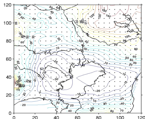
右図：ブーゲー異常図 (密度 2.2\text{g/cm}^3 ) 田中・他 (2005)
