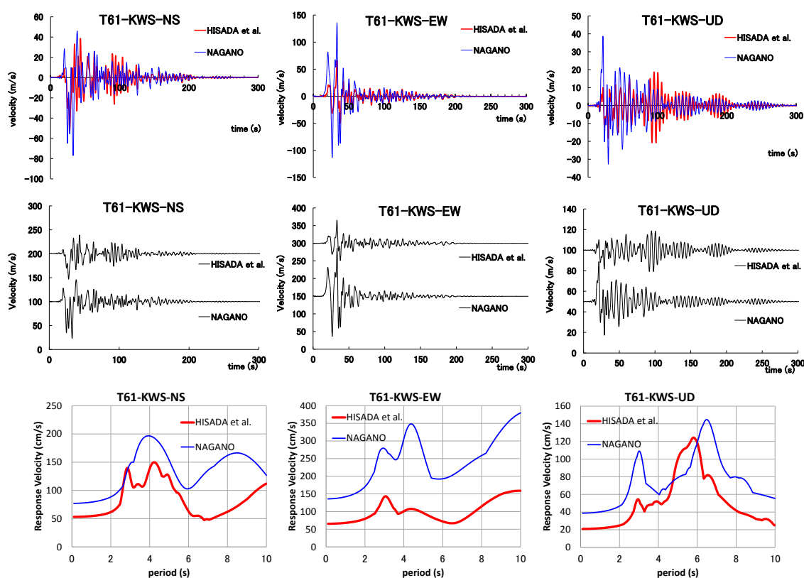
図 15 KWS の速度波形比較と速度応答スペクトル ( h=0.05 ) 比較
