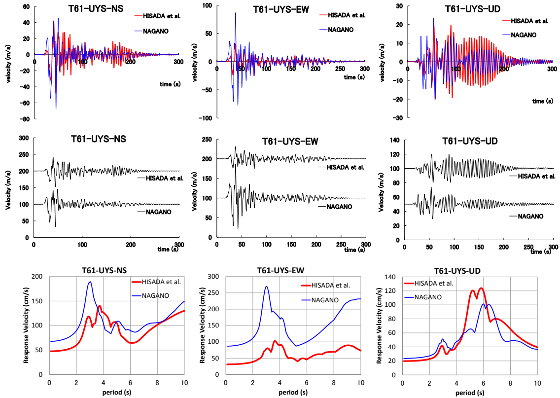
図 18 UYS の速度波形比較と速度応答スペクトル ( h=0.05 ) 比較
