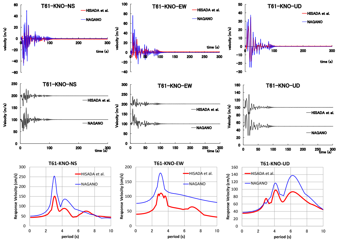
図6 KNOの速度波形比較と速度応答スペクトル ( h=0.05 ) 比較
