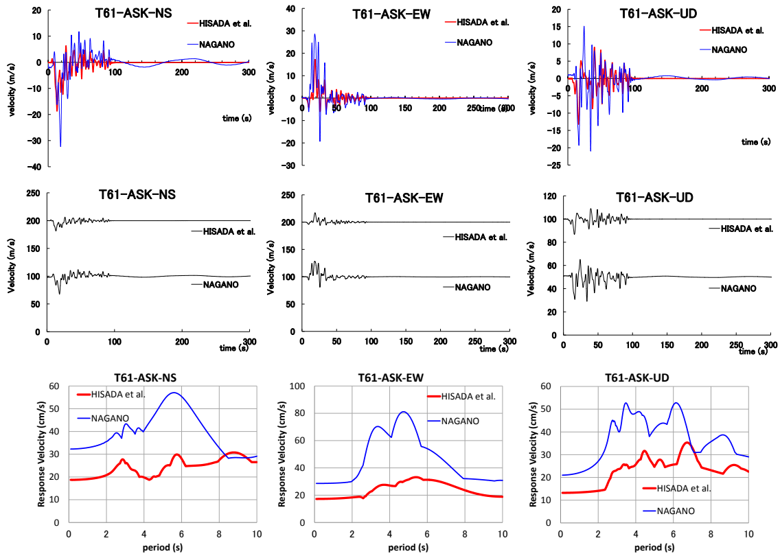
図9 ASKの速度波形比較と速度応答スペクトル ( h=0.05 ) 比較
