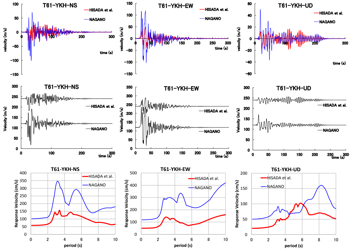
図 14 YKH の速度波形比較と速度応答スペクトル ( h=0.05 ) 比較
