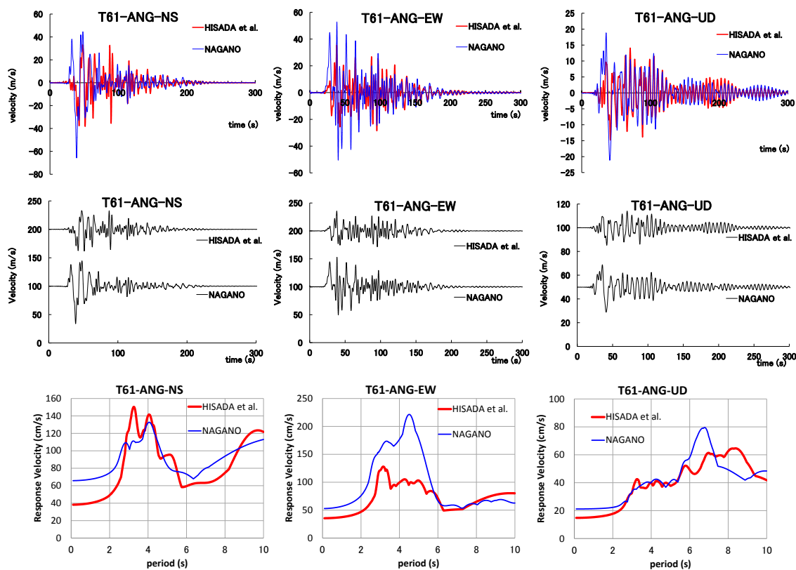
図 20 ANG の速度波形比較と速度応答スペクトル ( h=0.05 ) 比較
