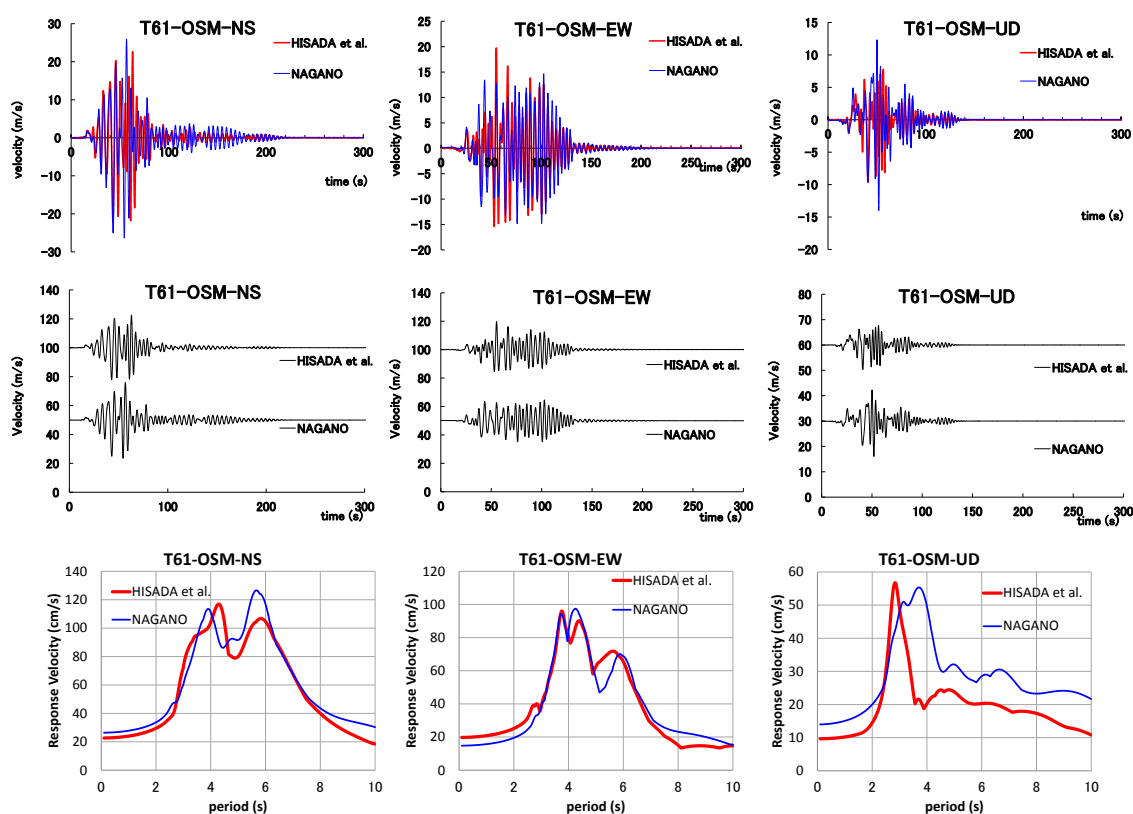
図3 OSM の速度波形比較と速度応答スペクトル ( h=0.05 ) 比較
