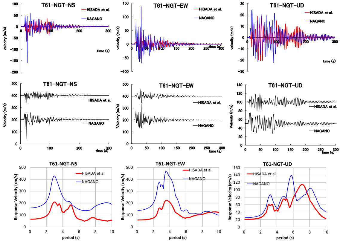
図8 NGTの速度波形比較と速度応答スペクトル (h=0.05) 比較
