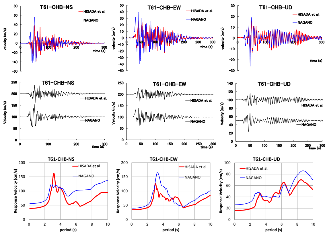
図 19 CHB の速度波形比較と速度応答スペクトル ( h=0.05 ) 比較
