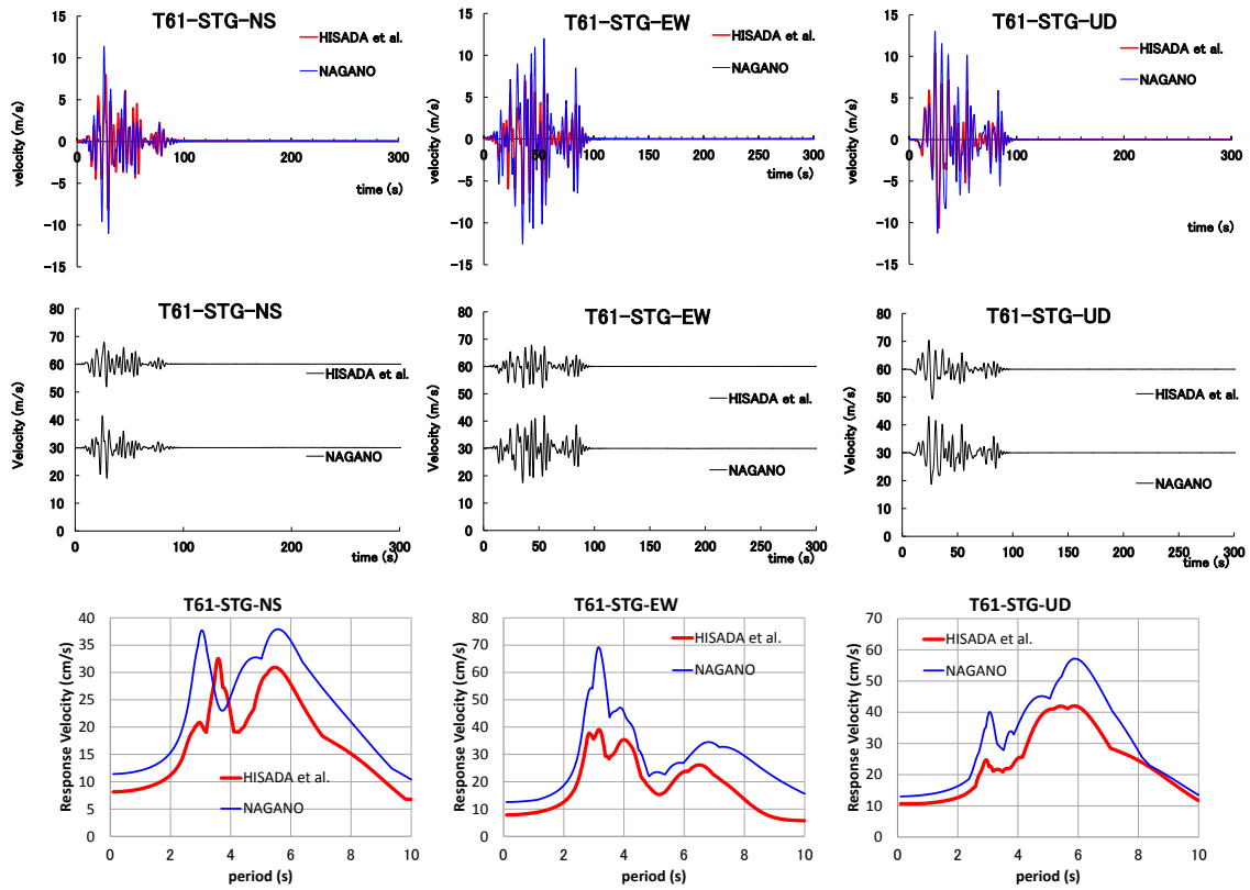
図5 STGの速度波形比較と速度応答スペクトル ( h=0.05 ) 比較
