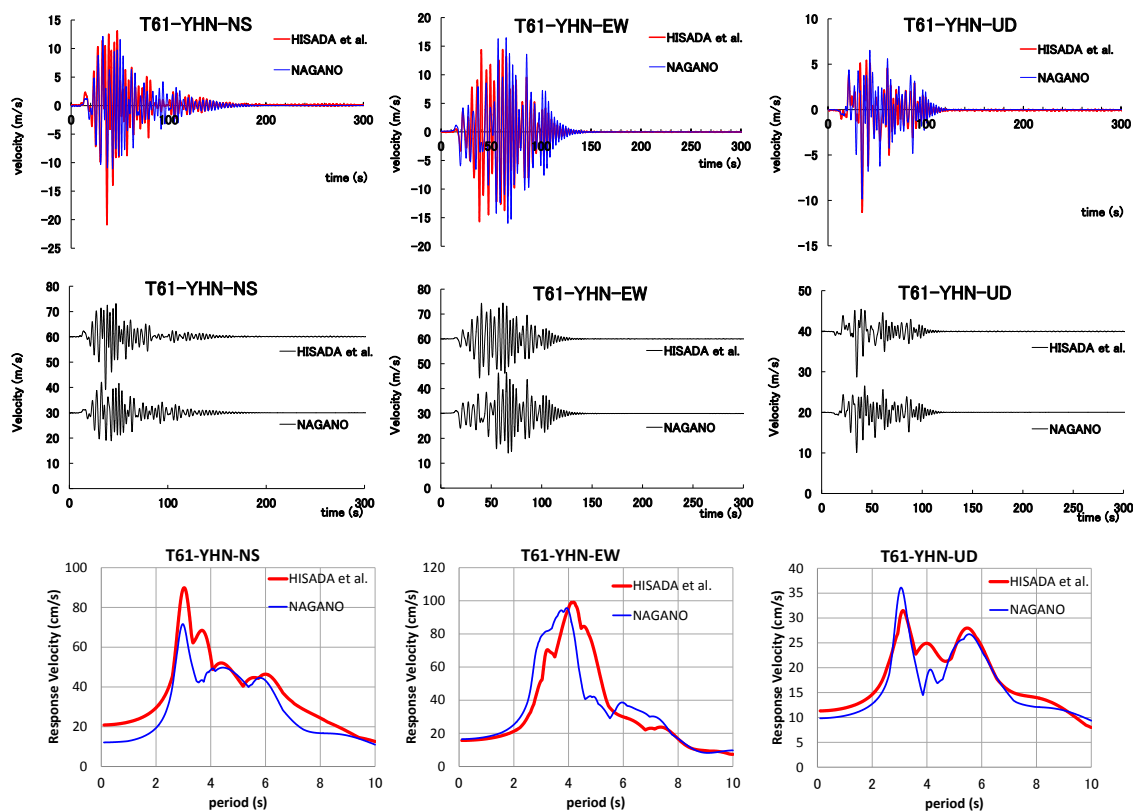
図4 YHN の速度波形比較と速度応答スペクトル ( h=0.05 ) 比較
