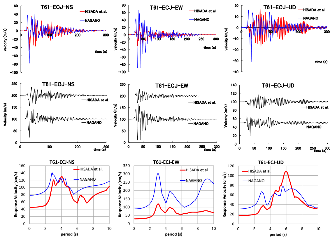
図 16 ECJ の速度波形比較と速度応答スペクトル ( h=0.05 ) 比較
