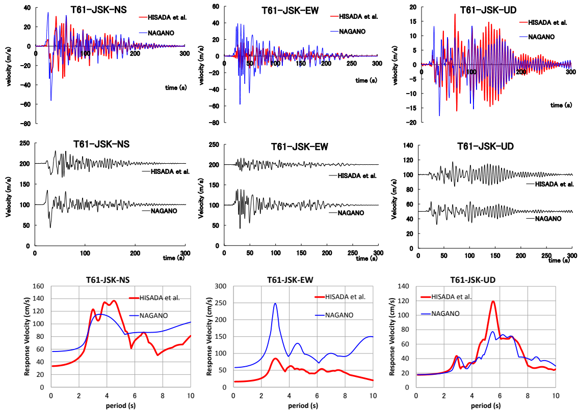
図 17 JSK の速度波形比較と速度応答スペクトル ( h=0.05 ) 比較
