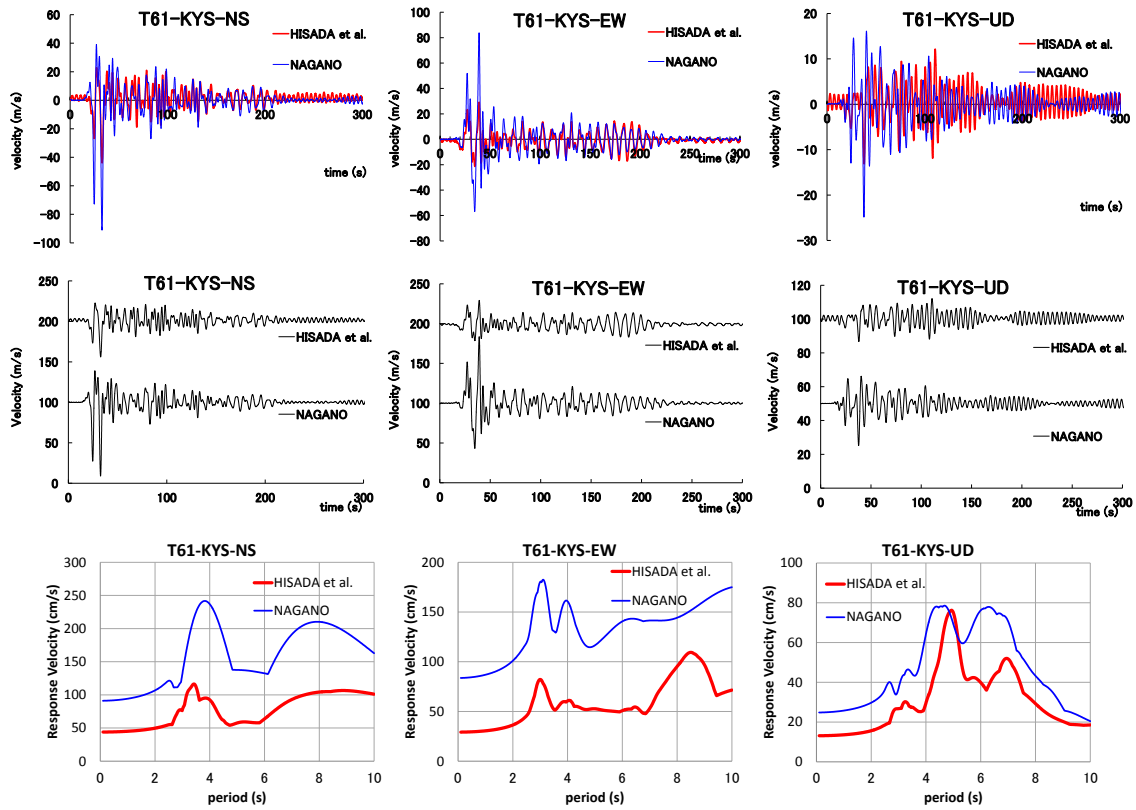
図 11 KYS の速度波形比較と速度応答スペクトル ( h=0.05 ) 比較
