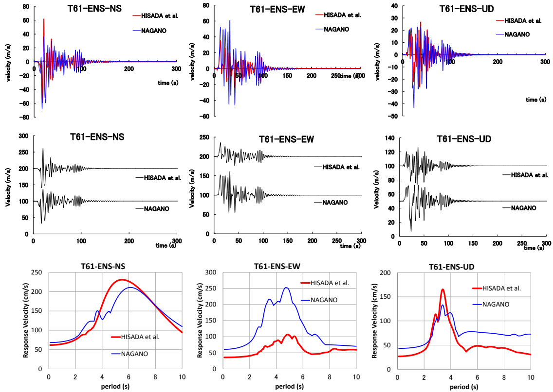
図 12 ENS の速度波形比較と速度応答スペクトル ( h=0.05 ) 比較
