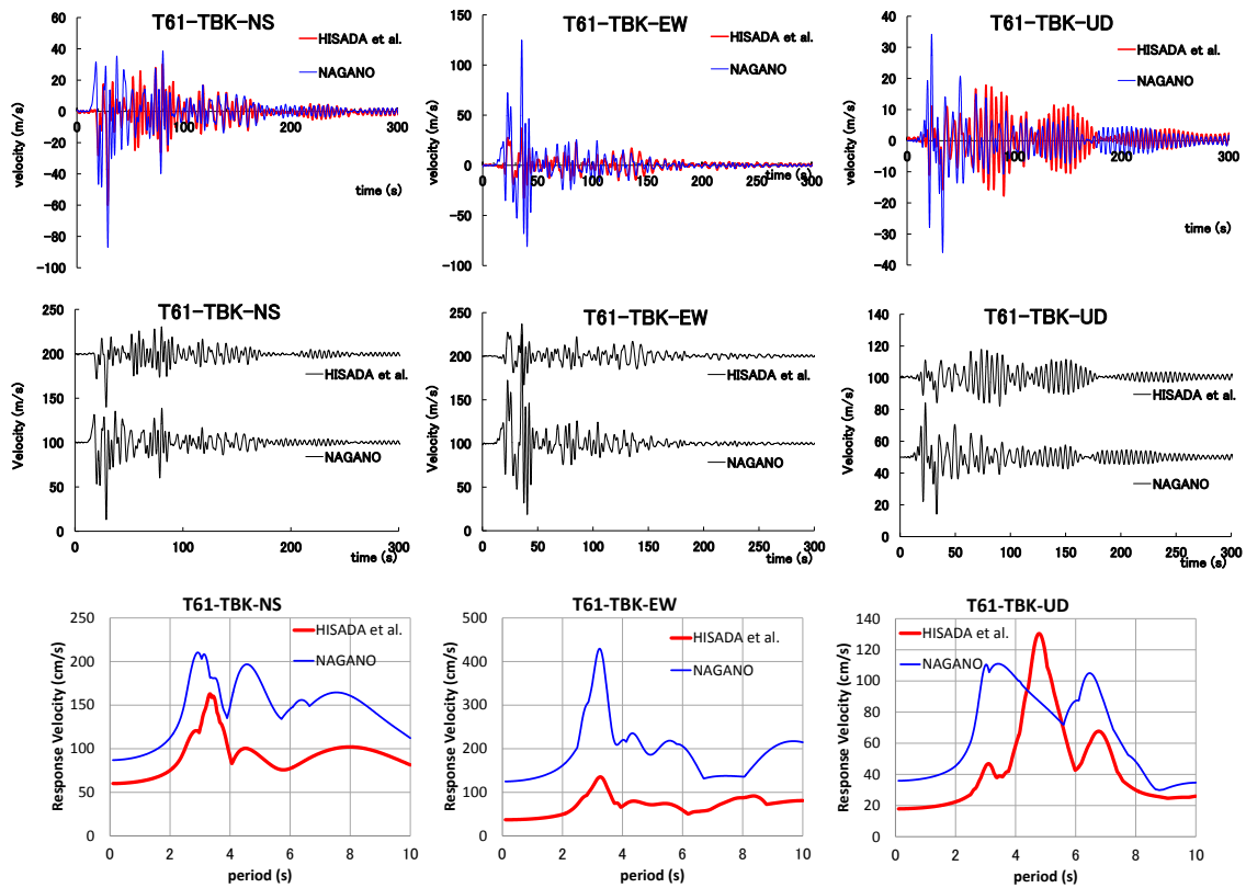
図10 TBKの速度波形比較と速度応答スペクトル ( h=0.05 ) 比較
