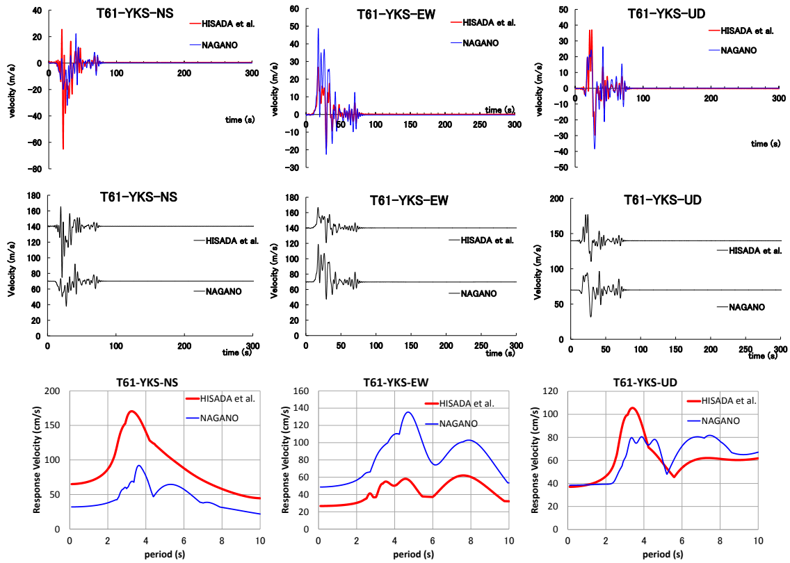
図 13 YKS の速度波形比較と速度応答スペクトル ( h=0.05 ) 比較
