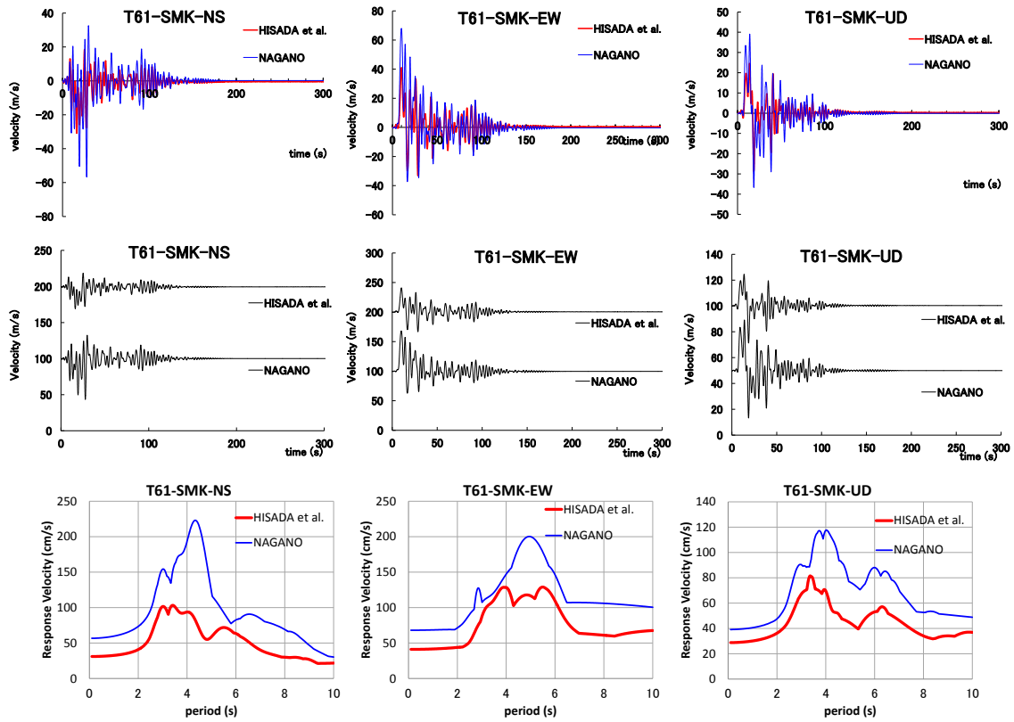
図7 SMKの速度波形比較と速度応答スペクトル (h=0.05) 比較
