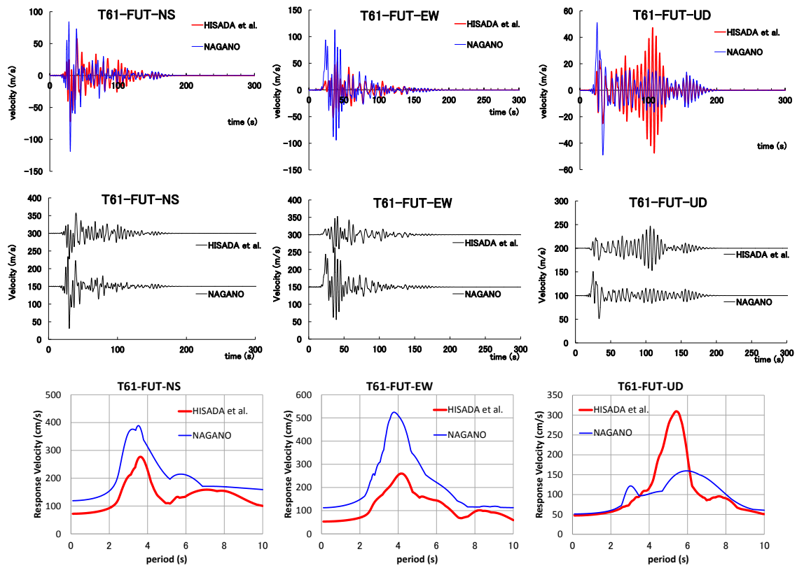
図 21 FUT の速度波形比較と速度応答スペクトル ( h=0.05 ) 比較
