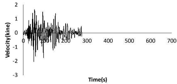
10901E02-B3F N059E-VEL-FIL
