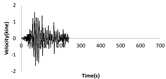
10401E02-100 N080E-VEL-FIL
