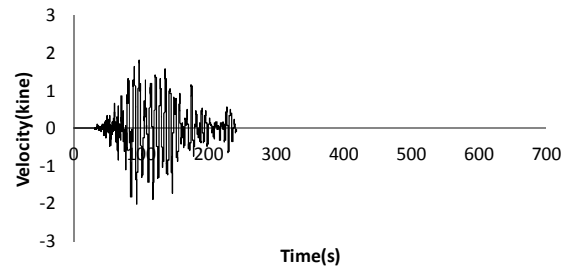
11303E02-100 N354E-VEL-FIL
