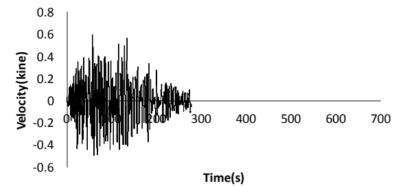
10901E02-B3F UD-VEL-FIL
