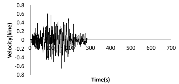
10701E02-052 UD-VEL-FIL
