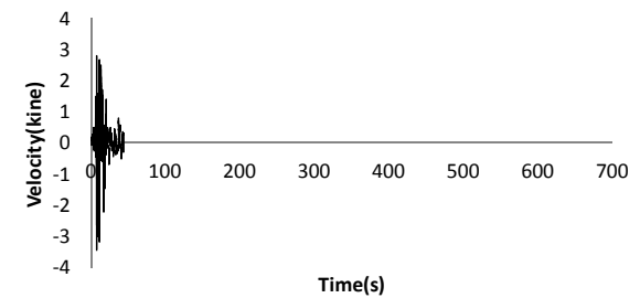
80241E02-GL0 N270E-VEL-FIL
