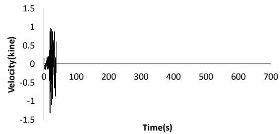
10406E02-GL0 N090E-VEL-FIL
