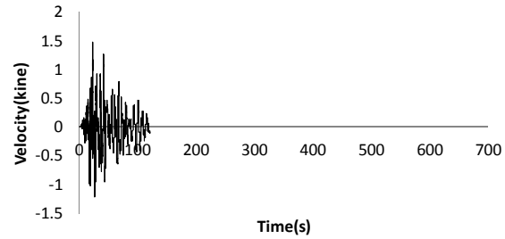
80205E02-GL0 N000E-VEL-FIL
