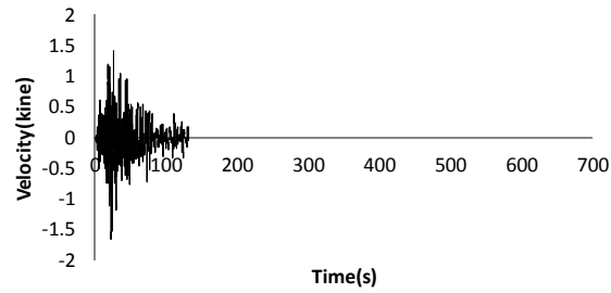
80206E02-GL0 UD-VEL-FIL
