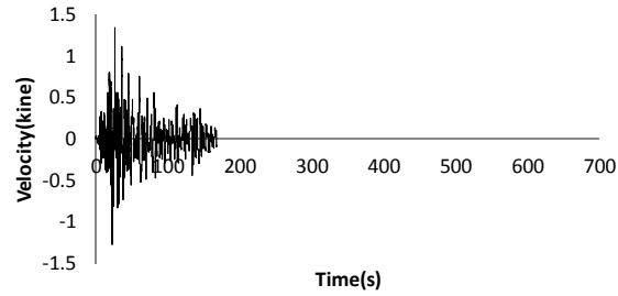
80207E02-GL0 UD-VEL-FIL
