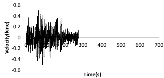
10408E02-047 UD-VEL-FIL
