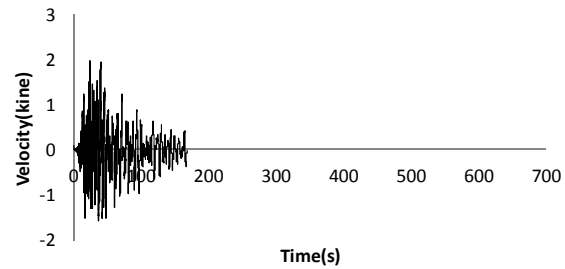
80207E02-GL0 N000E-VEL-FIL
