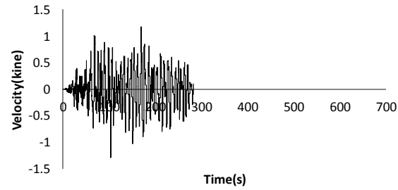
10701E02-052 N090E-VEL-FIL
