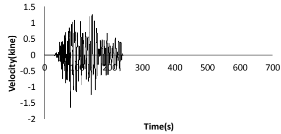
11303E02-100 N084E-VEL-FIL
