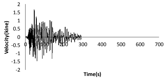
80301E02-B1FN090E-VEL
