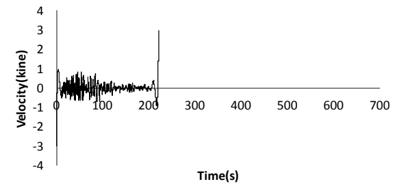
10501E02-075 UP-VEL-FIL
