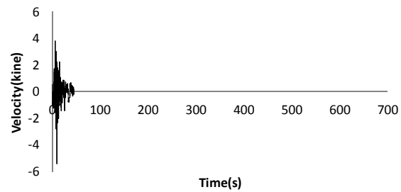
50101E02-B1F NS-VEL-FIL
