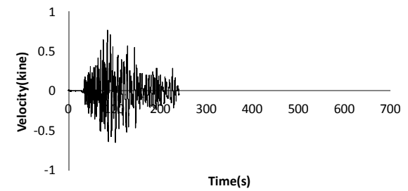
11303E02-100 UP-VEL-FIL
