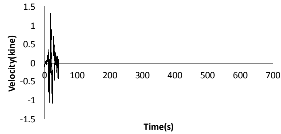
10405E02-059 N090E-VEL-FIL
