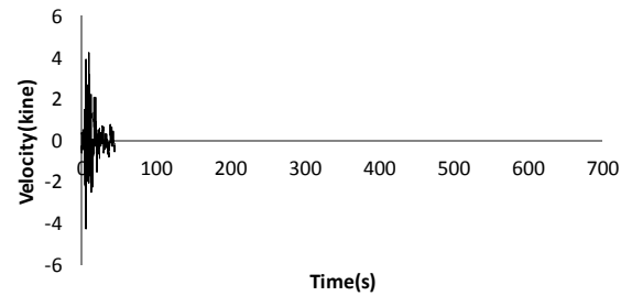
50101E02-B1F EW-VEL-FIL
