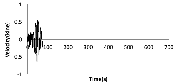
10803E02-B1F N356E-VEL-FIL
