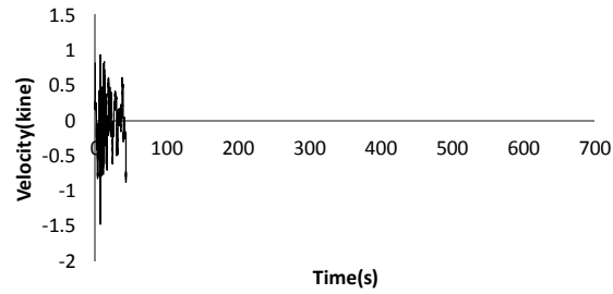
80241E02-GL0 UD-VEL-FIL
