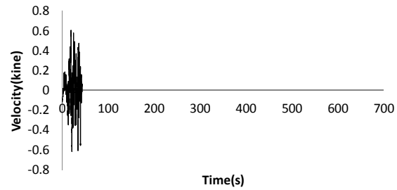
10405E02-059 N000E-VEL-FIL
