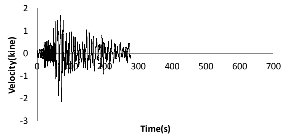
10901E02-B3F N329E-VEL-FIL
