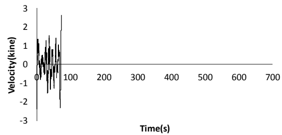
10803E02-B1F N086E-VEL-FIL
