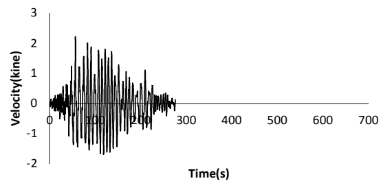
10408E02-047 N000E-VEL-FIL
