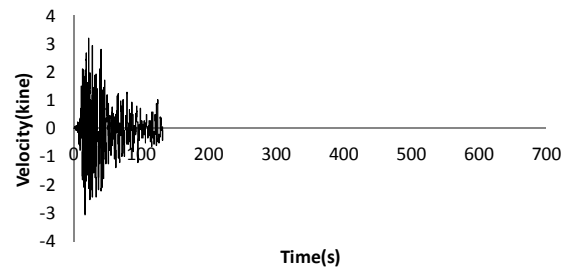
80206E02-GL0 N000E-VEL-FIL
