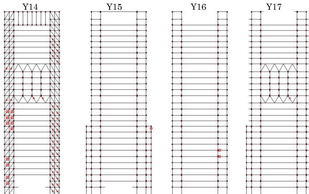
Ai-EW 層間変形角 1/50
