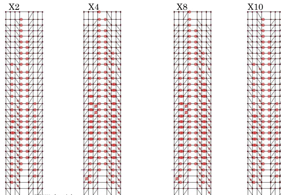
Ai-NS 層間変形角 1/50
