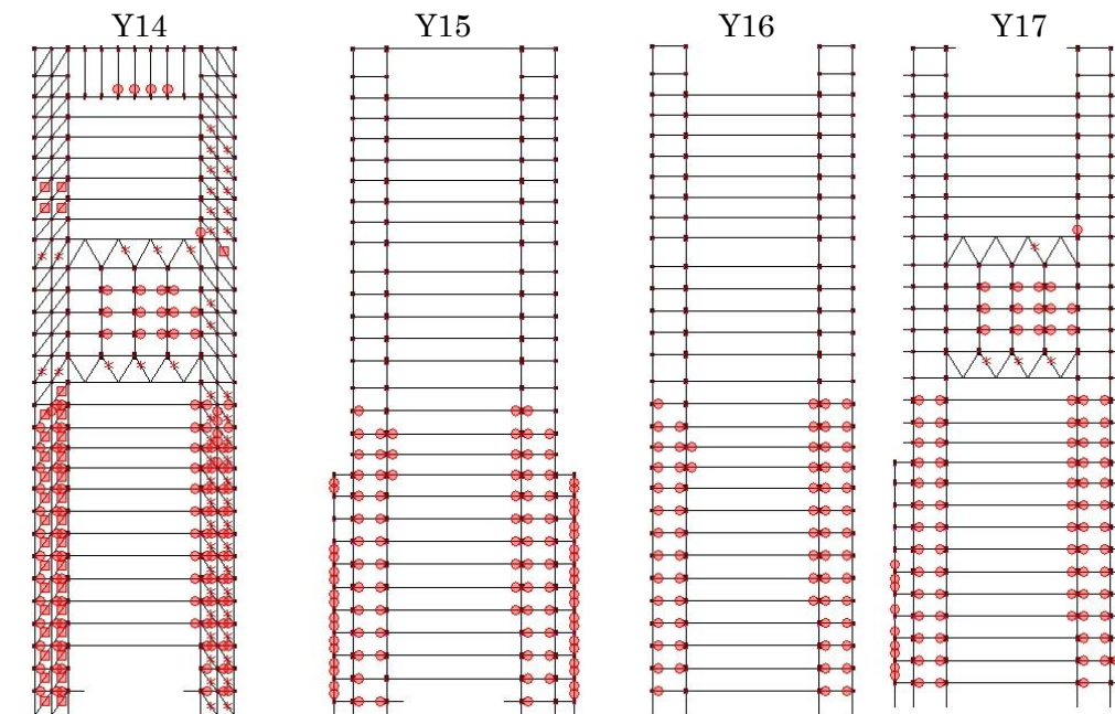
Ai-EW 層間変形角 1/50
