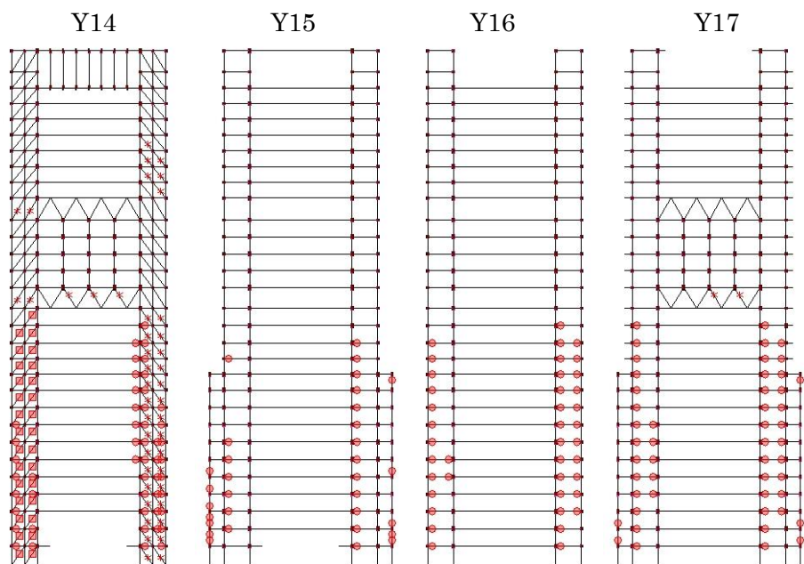
1 次モード EW 層間変形角 1/75
