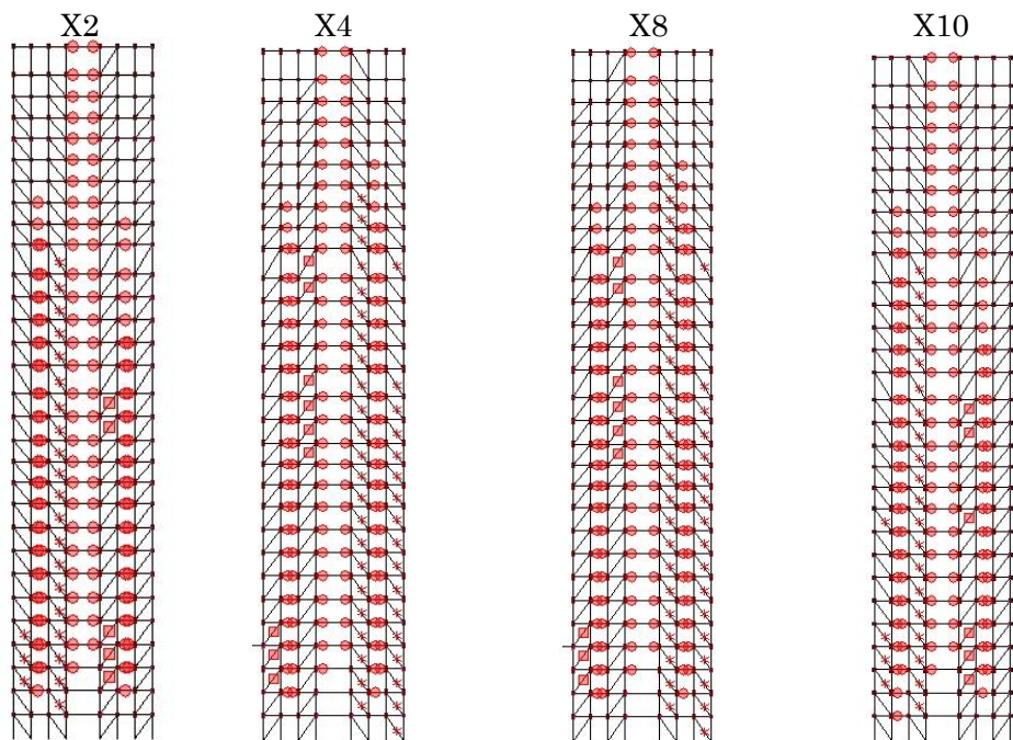
Ai-NS 層間変形角 1/75
