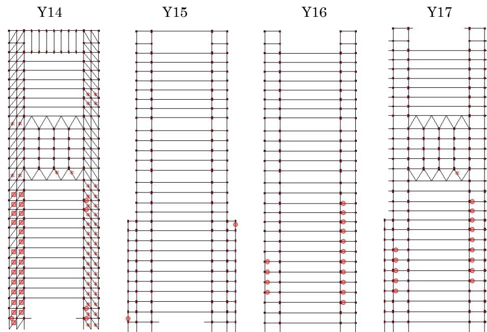
1 次モード EW 層間変形角 1/50
