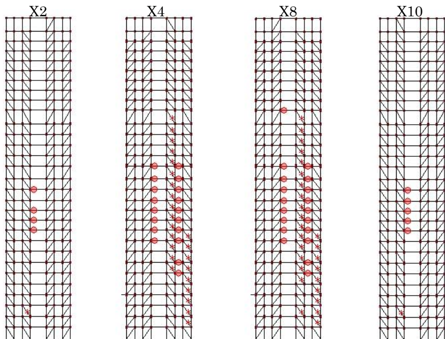
1 次モード NS 層間変形角 1/75
