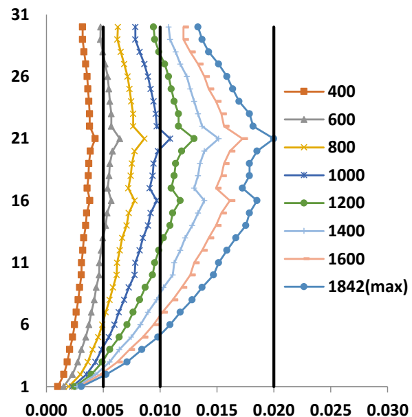
階 告示平均-NS最大層間変形角
