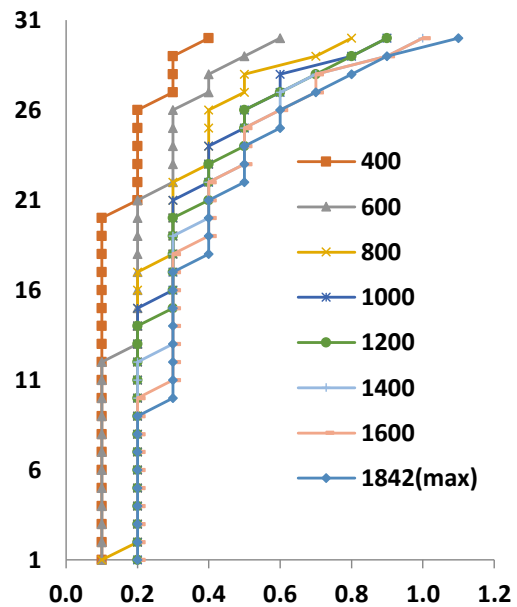
階 告示平均-NS層せん断力係数
