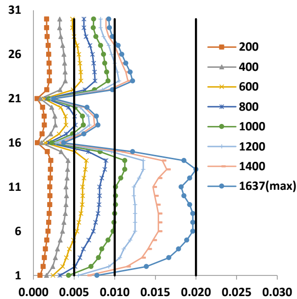
階 告示平均-EW最大層間変形角
