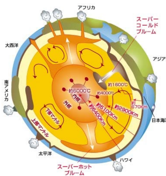
図2 地球の内部構造 ( http://www.jamstec.go.jp/jamstec-j/enlight/umihoshi/learning/3_2200.html )
