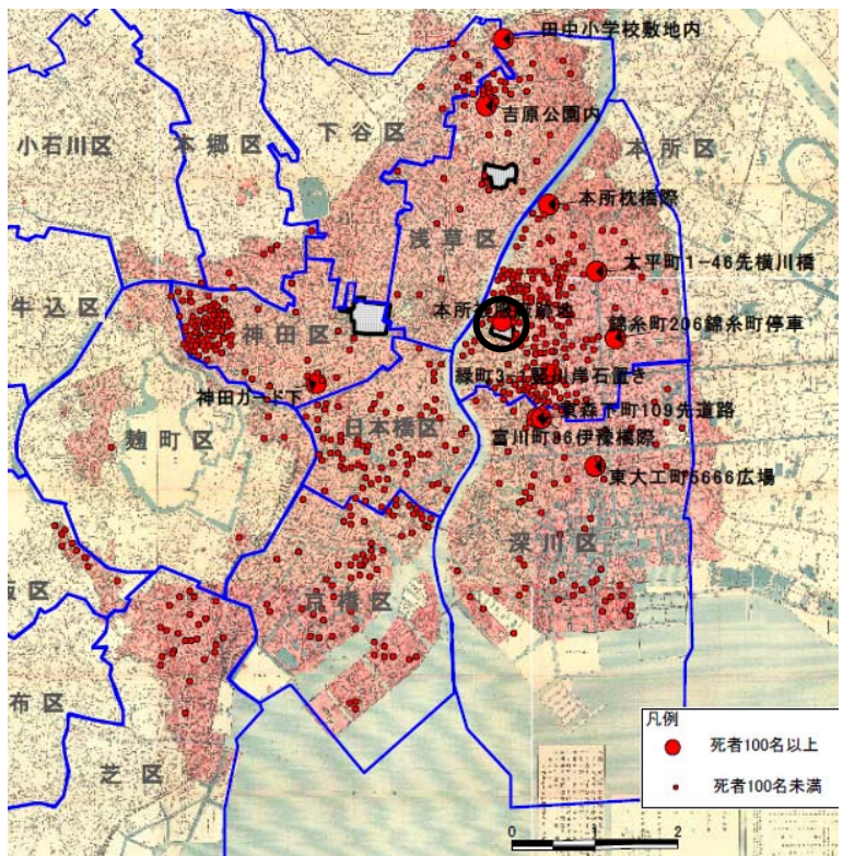
図 10 関東地震による東京市の延焼地域と死者分布（中央防災会議、災害教訓の継承に関する専門調査会報告書）
