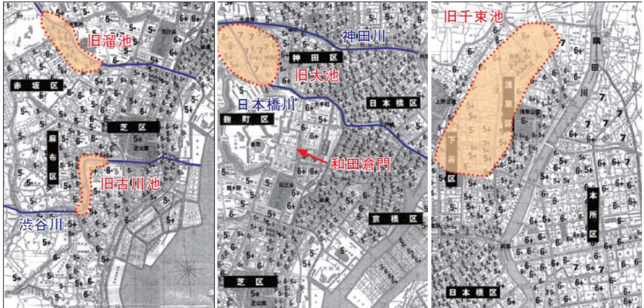
図 1 1 関東大震災における東京市の埋め立て地盤と震度の関係東京市の住宅全潰率（関東地質調査業協会、東京の地名と地形、 http://www.kanto-geo.or.jp/tokyo_note/No39_2.pdf ）
