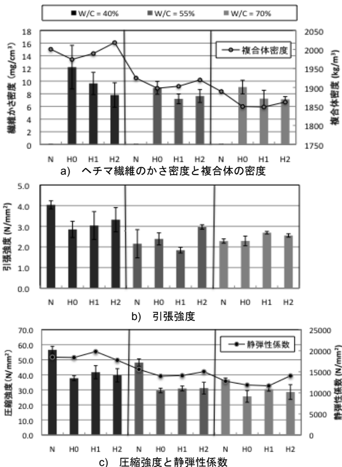
図8 無機有機複合体の基礎物性
