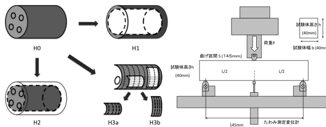
図2 有機物骨格 切断モデル
