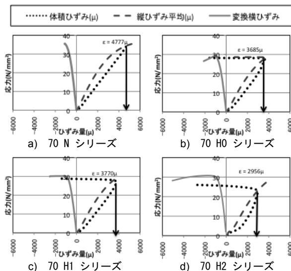
図10 破壊臨界ひずみ特性 (w/c = 70%)
